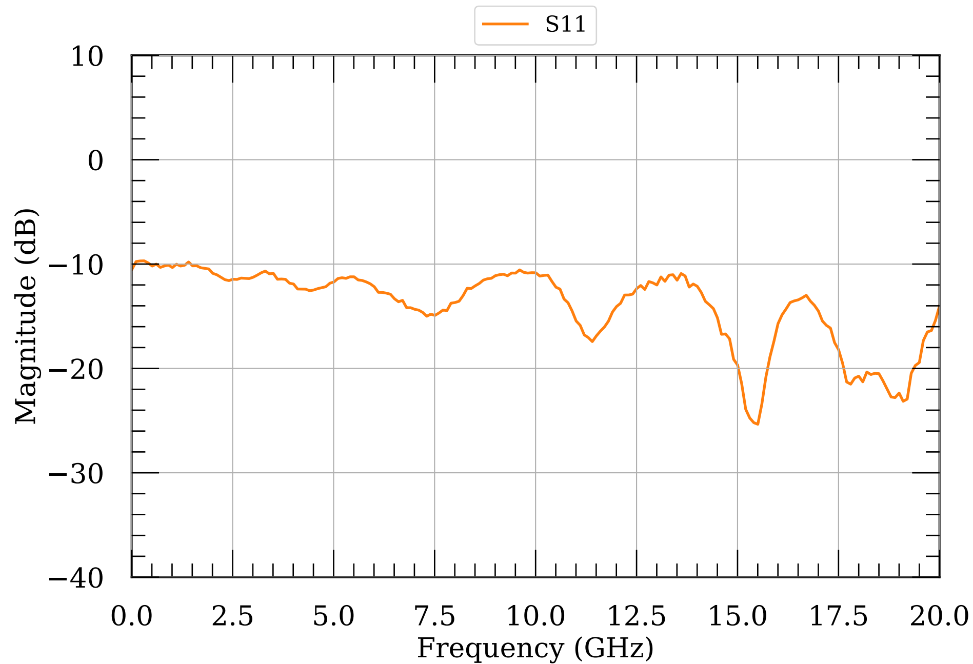
LNA S-params module075
